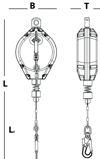
IKV 33 (ANSI Z.359.1-2007; CSA Z259.12-2011) mit Fallanzeiger
